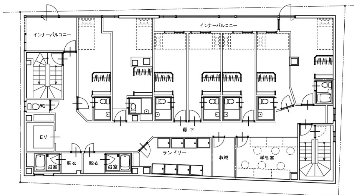
3 階平面図
