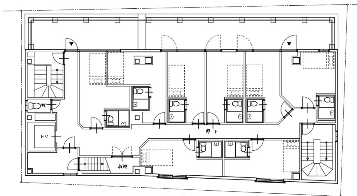
5 階平面図
