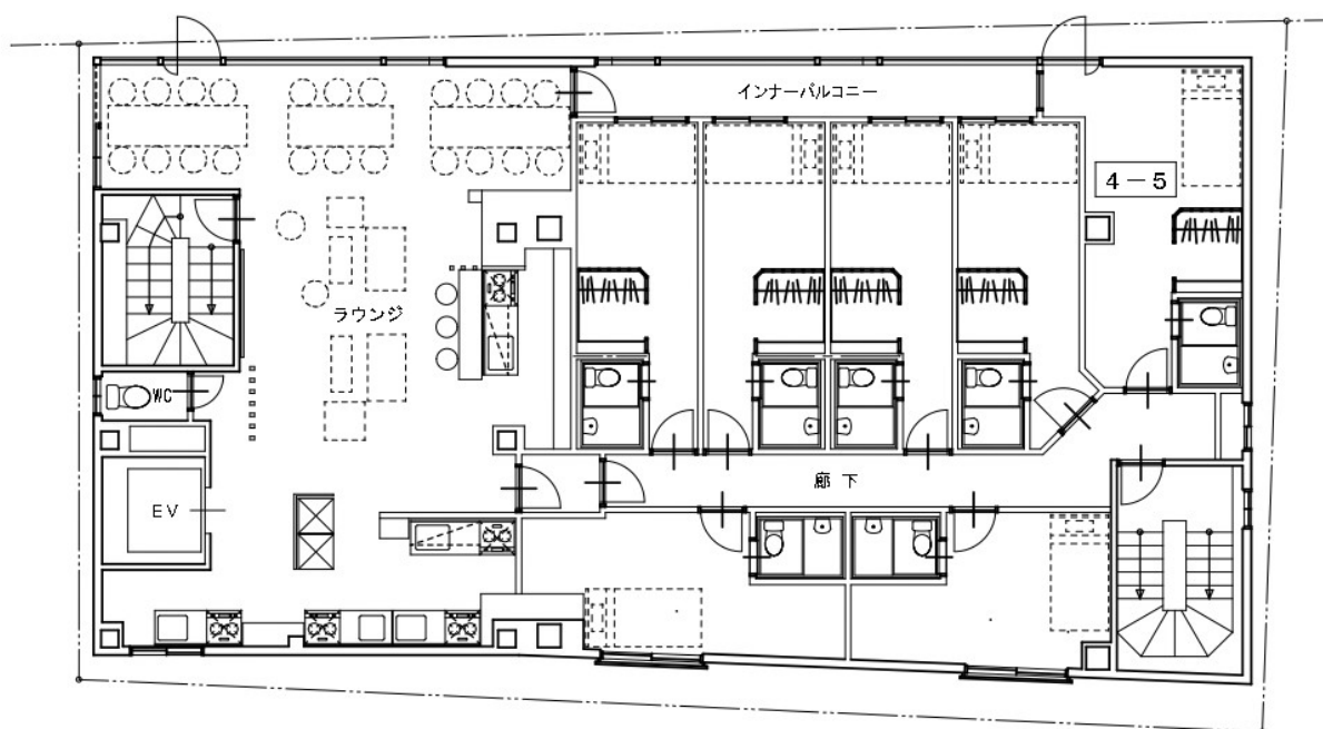
4 階平面図
