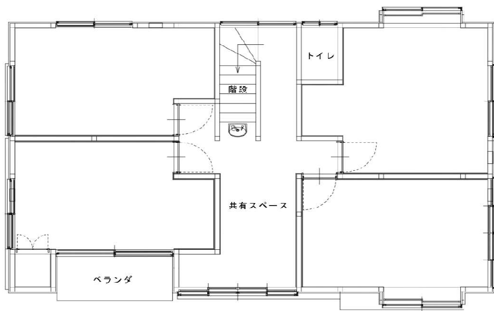
2 階平面図
