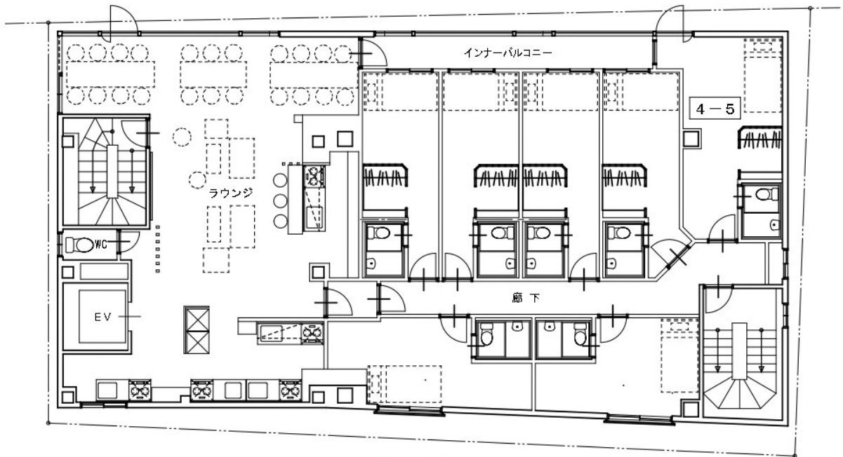
4階平面図
