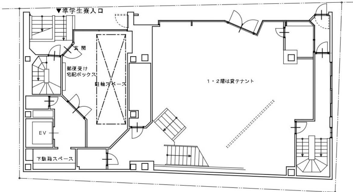
1階平面図
