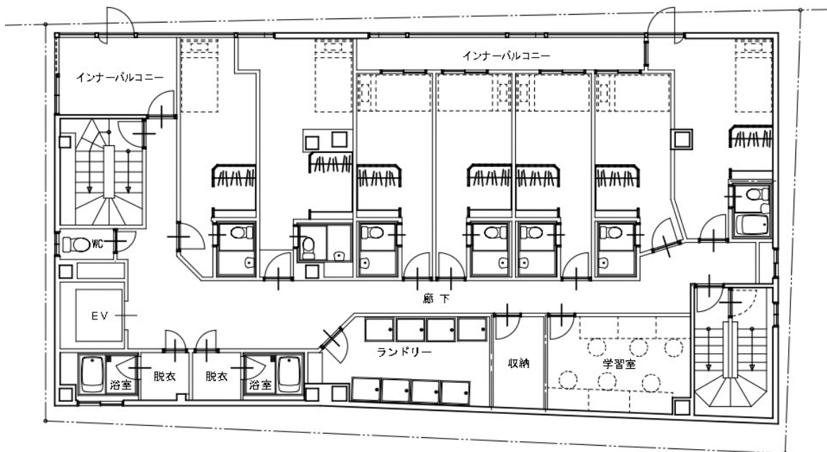
3階平面図
