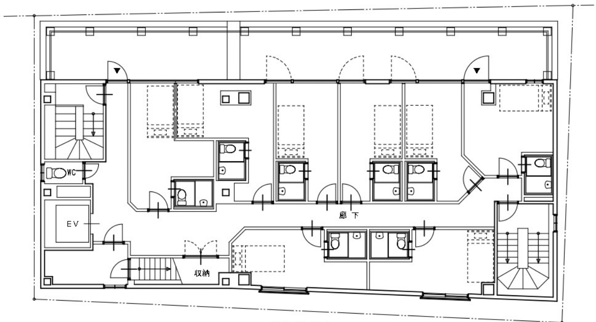
5階平面図
