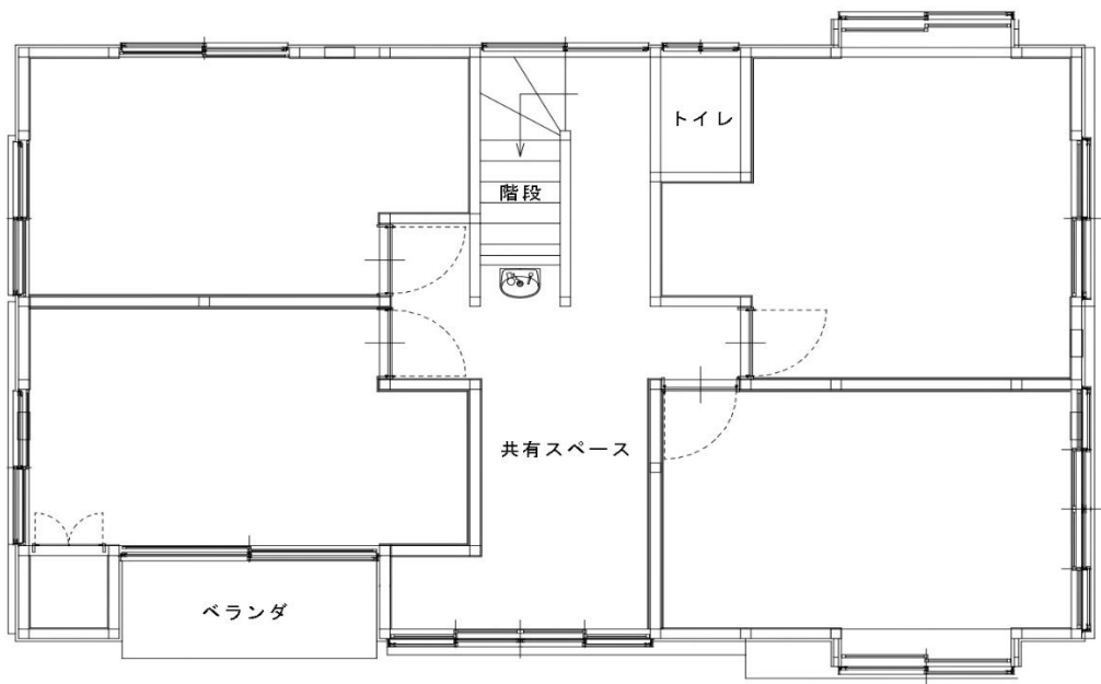
2階平面図
