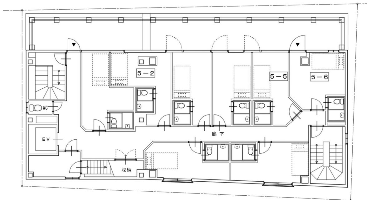
5階平面図
