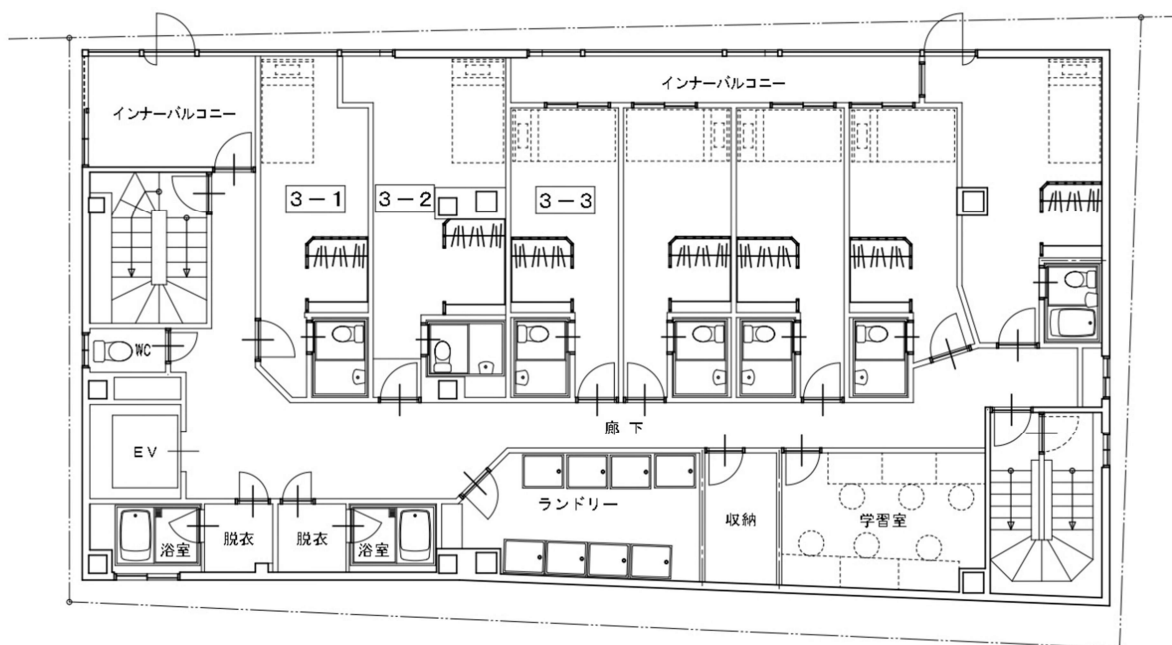
3 階平面図
