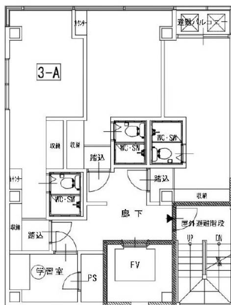
3階 平面図
