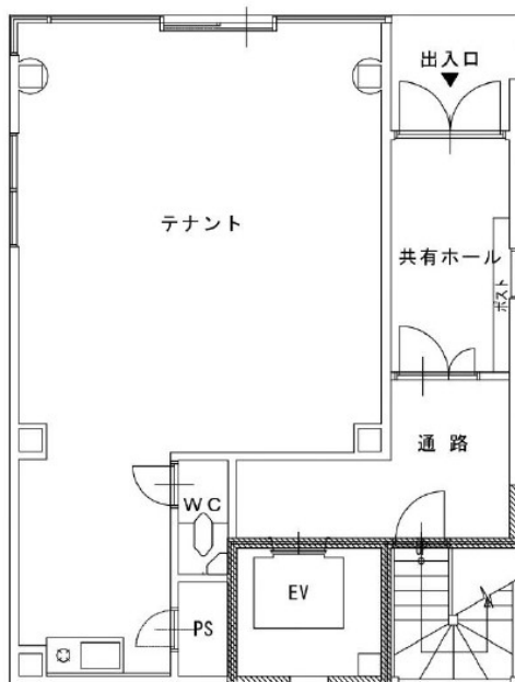
1階 平面図
