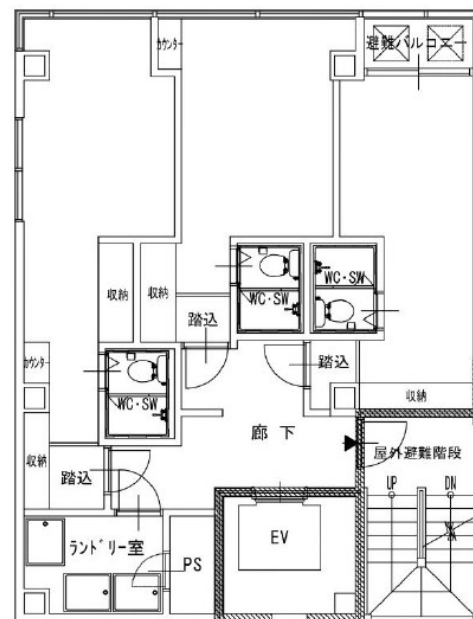
2階 平面図
