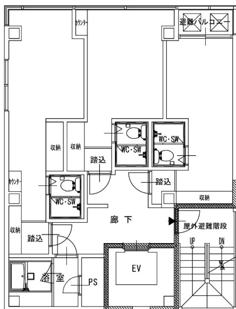
5 階 平面図
