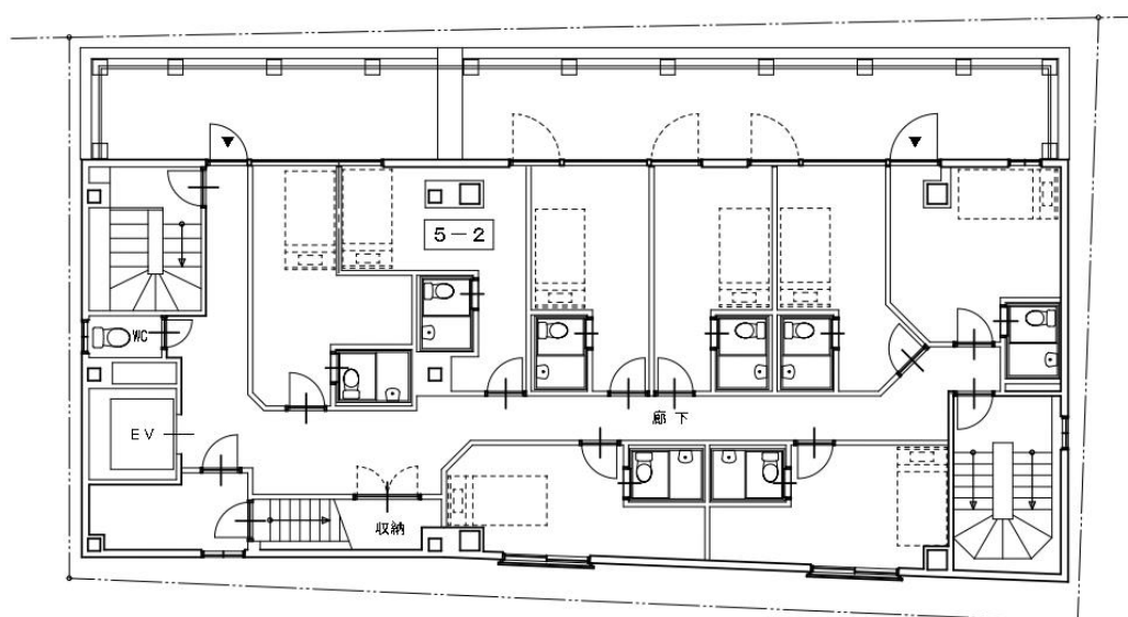
5 階平面図
