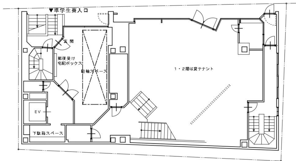
1 階平面図
