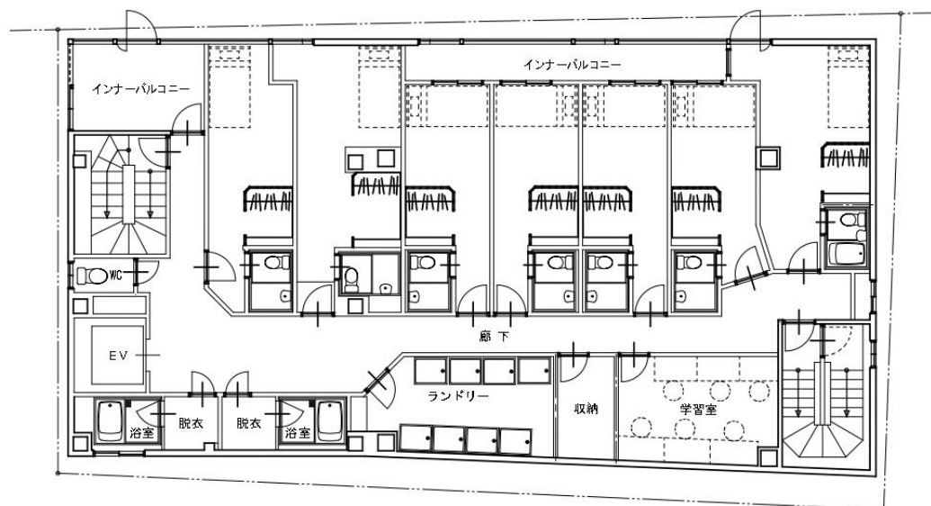
3 階平面図
