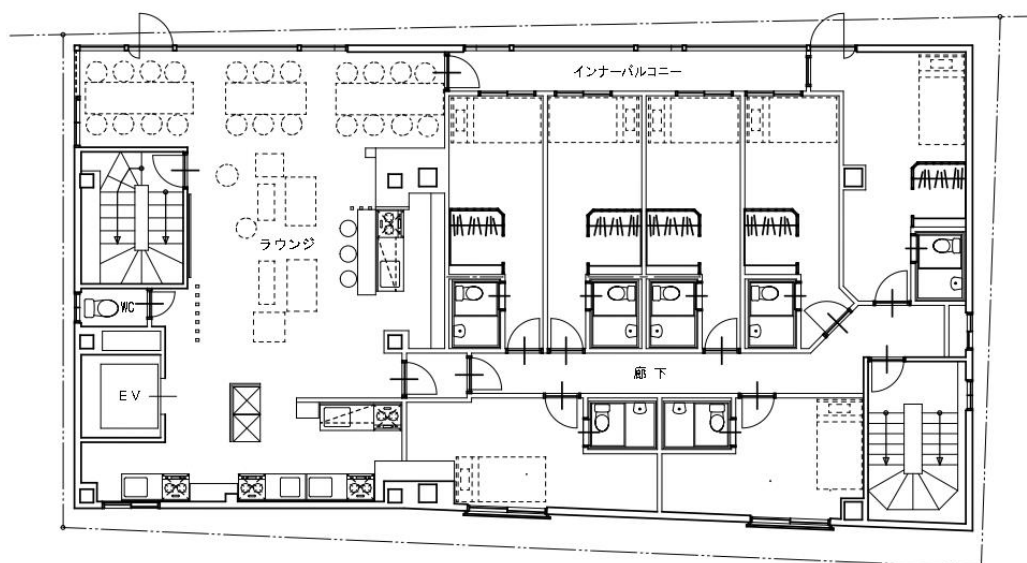
4 階平面図
