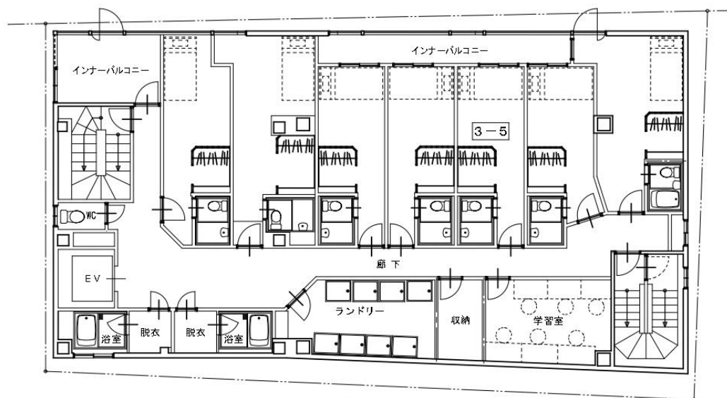
3階平面図
