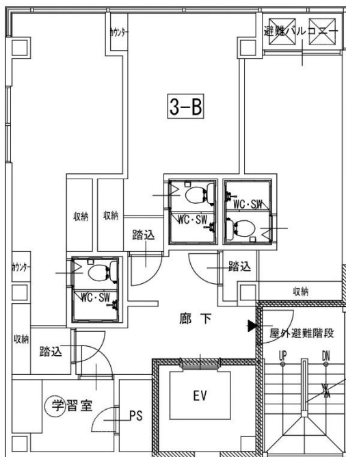
3階 平面図
