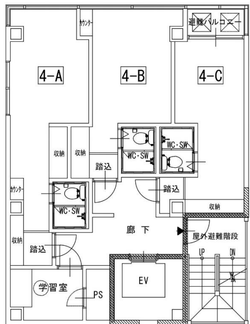
4階 平面図
