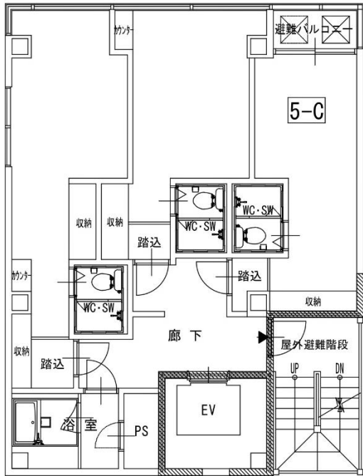
5階 平面図
