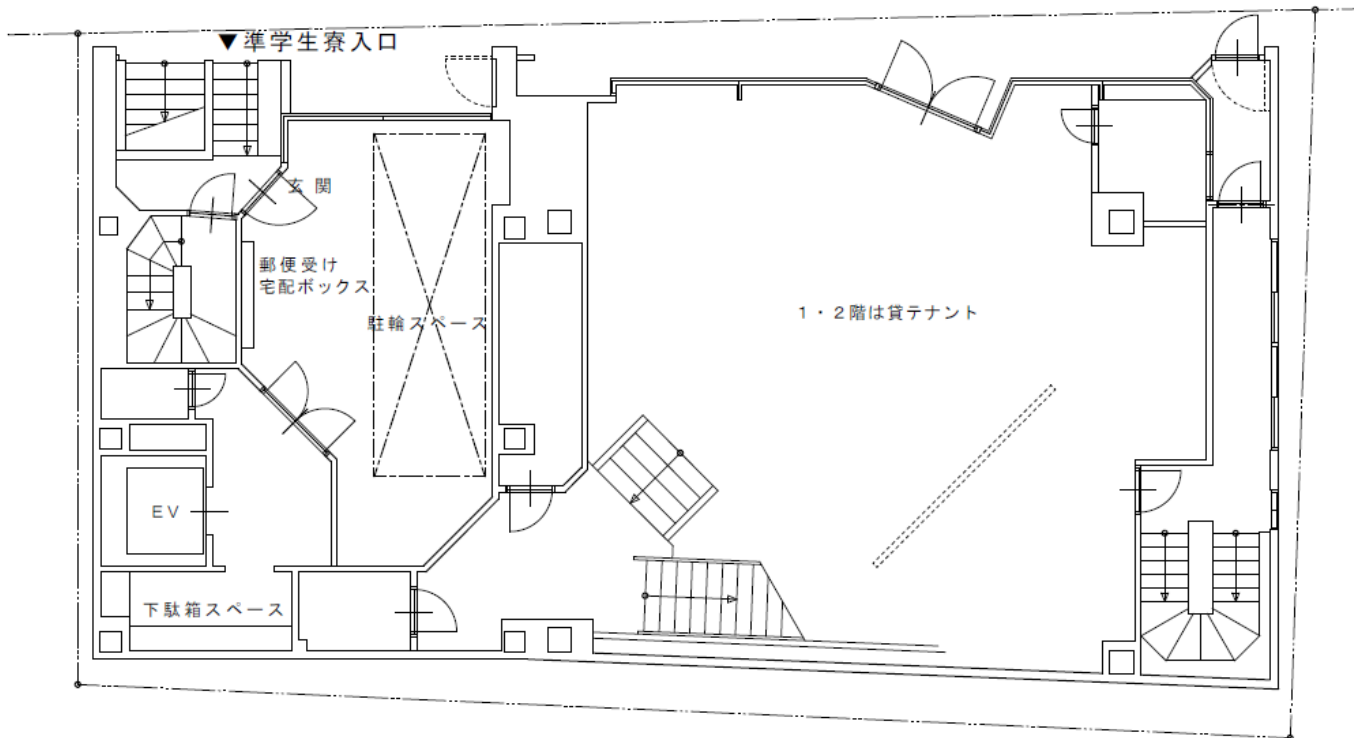
1階平面図
