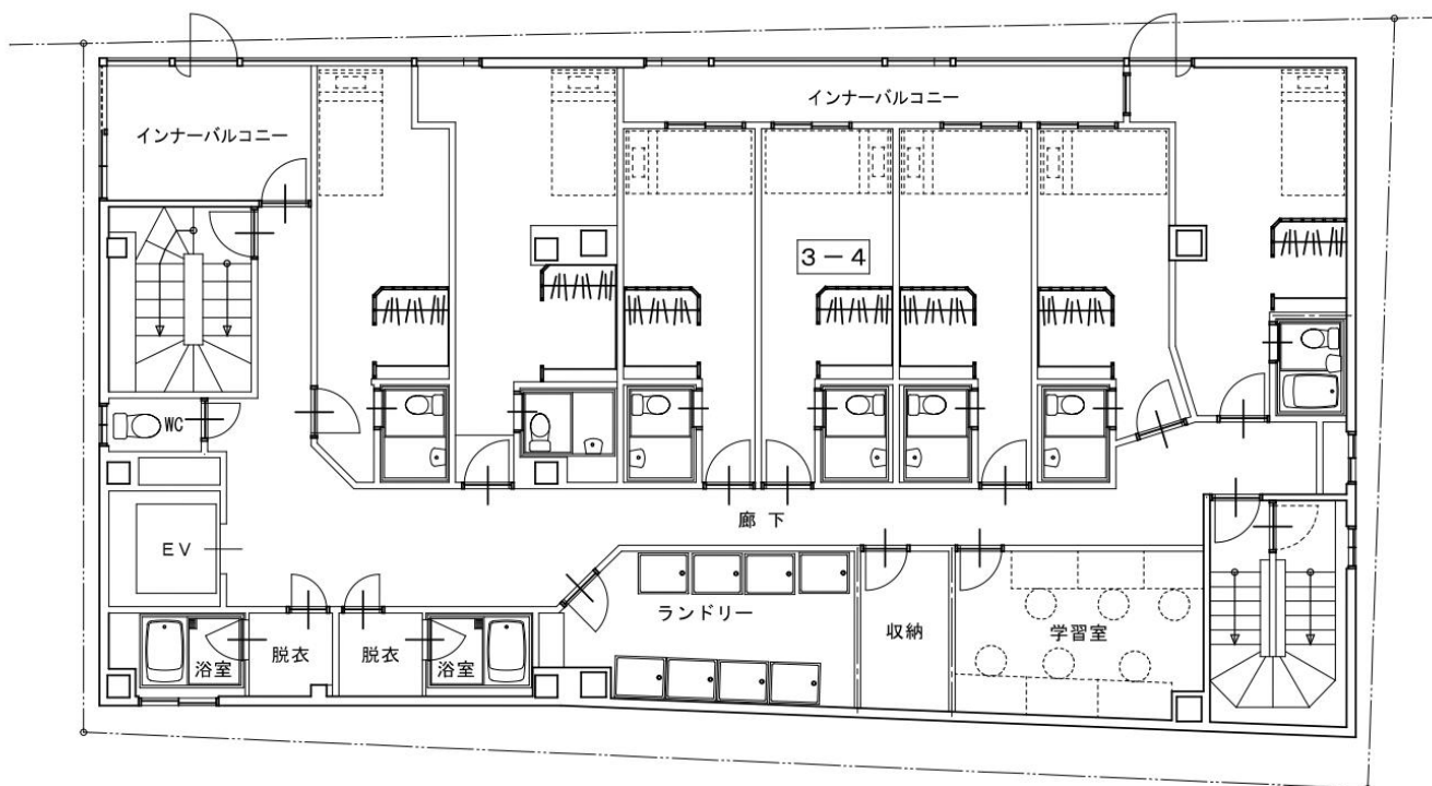
3階平面図
