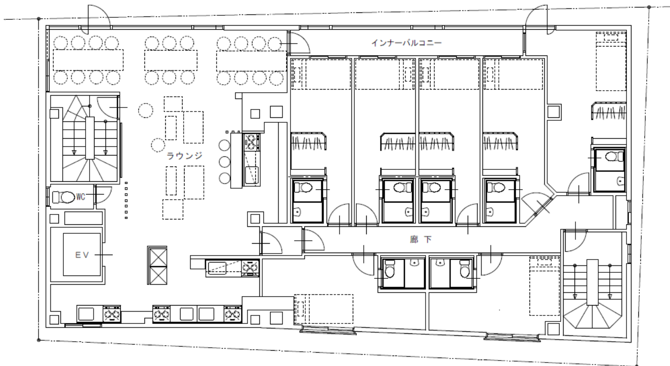
4階平面図
