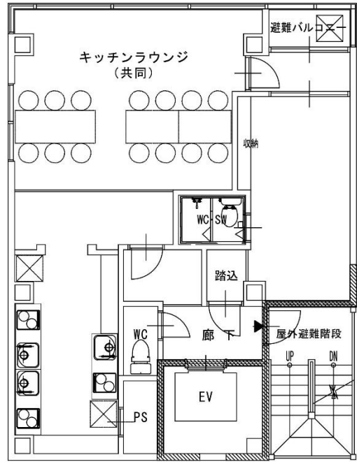
7階 平面図
