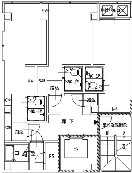
5階 平面図
