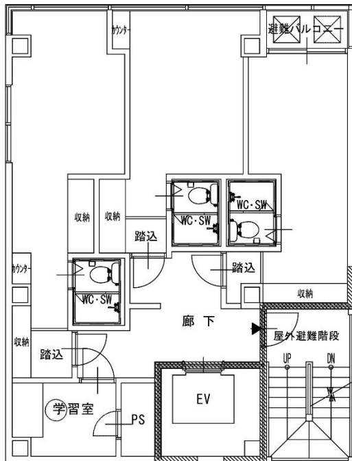
3階 平面図
