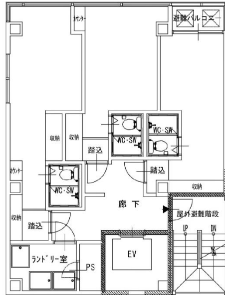
2階 平面図
