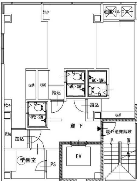
3階 平面図
