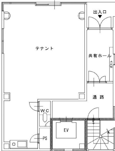
1階 平面図
