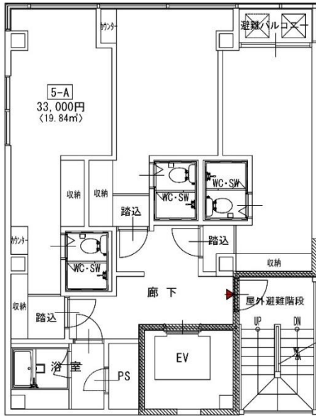
5階 平面図
