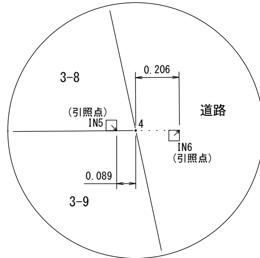
拡大図B 1/25
