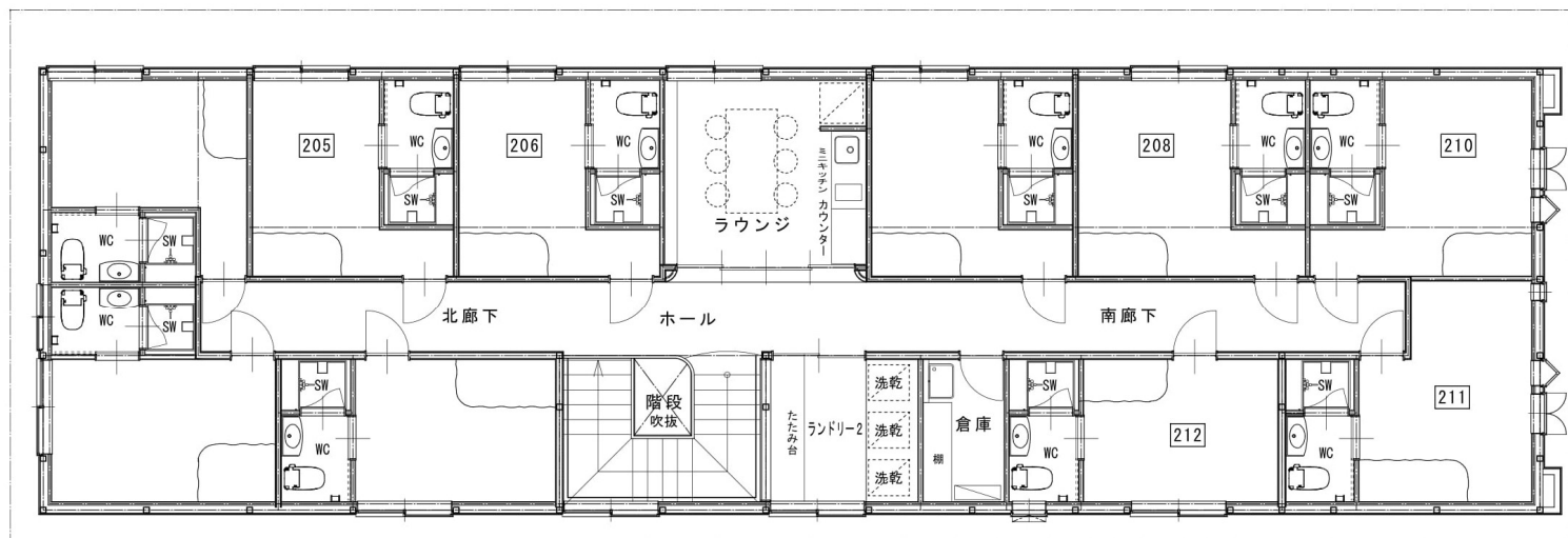
2階平面図
