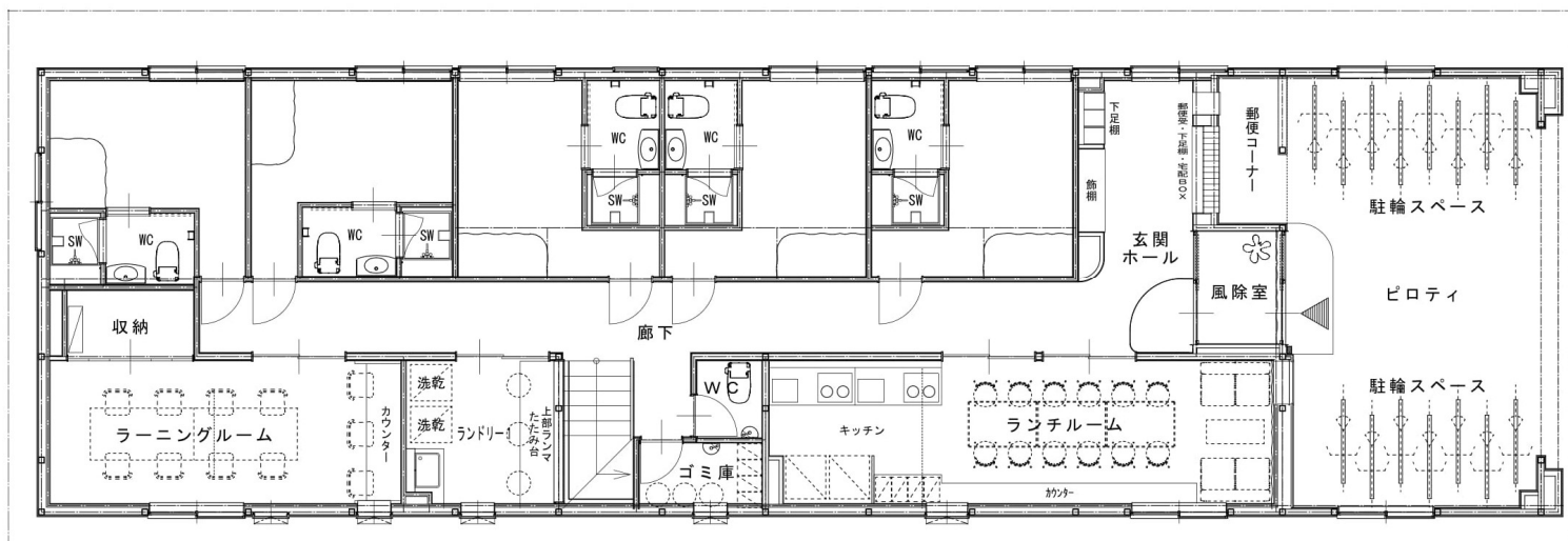
1階平面図
