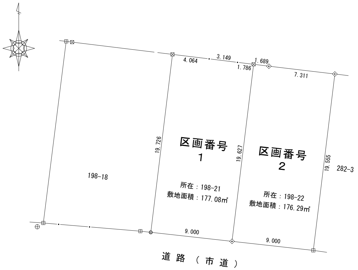
敷地平面図 (1/250)
